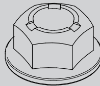
6x Nut, SRF 1/2-13 USS 99-SF08
